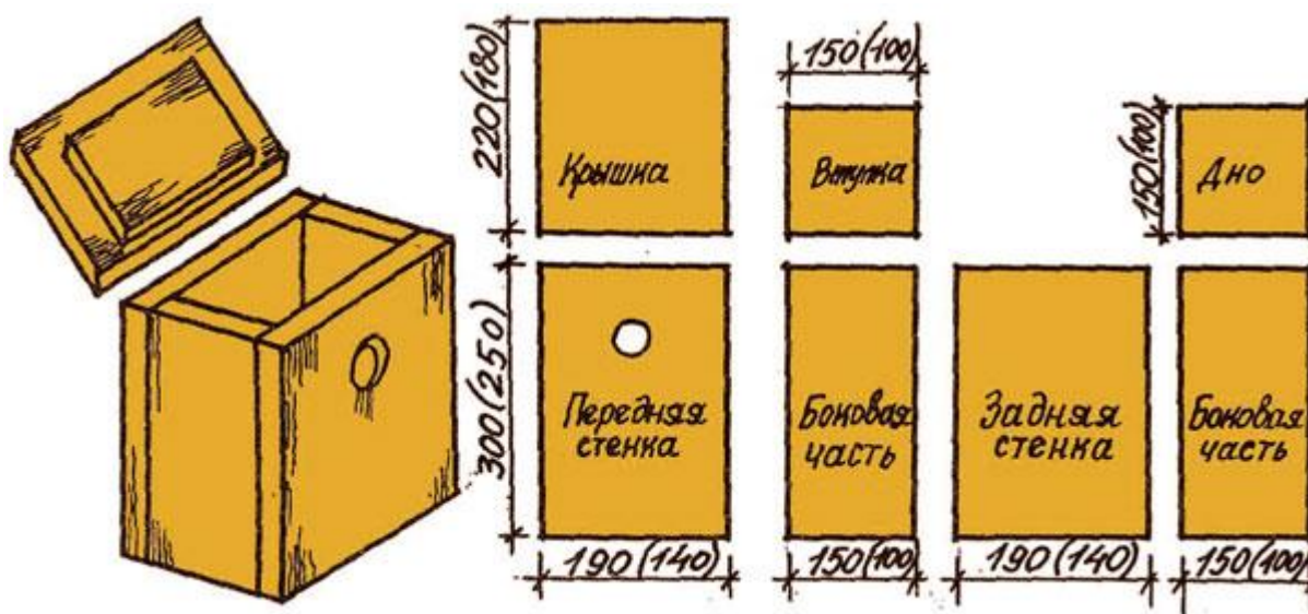
Рисунок 1. Размеры дощечек для изготовления скворечника
